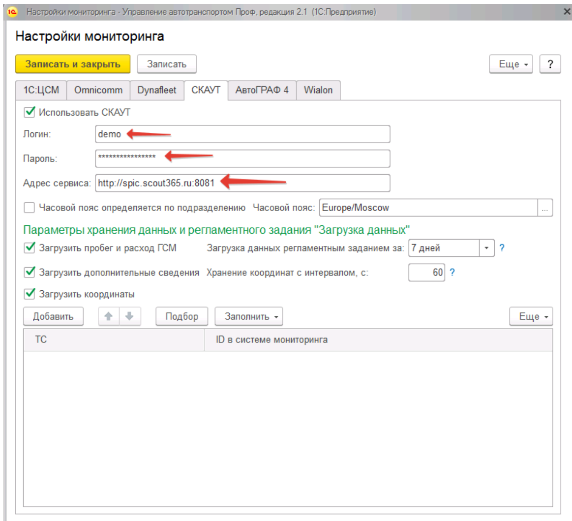
Рисунок 3 — Настройки мониторинга
